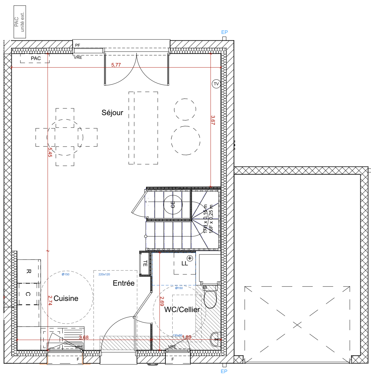
PLAN RdC
