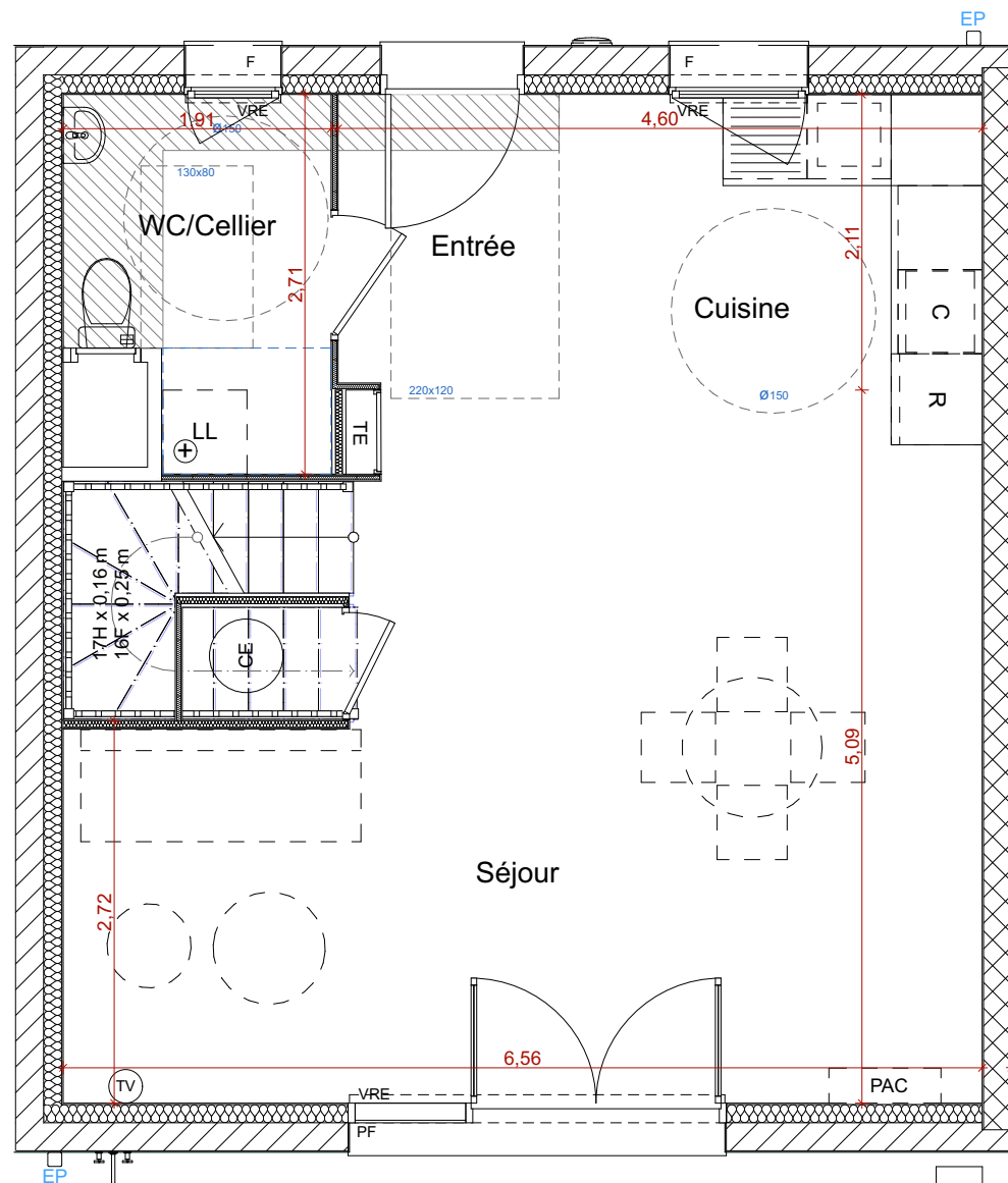
PLAN RdC
