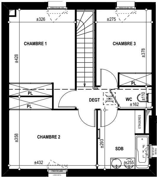
PLAN du NIVEAU R+1
