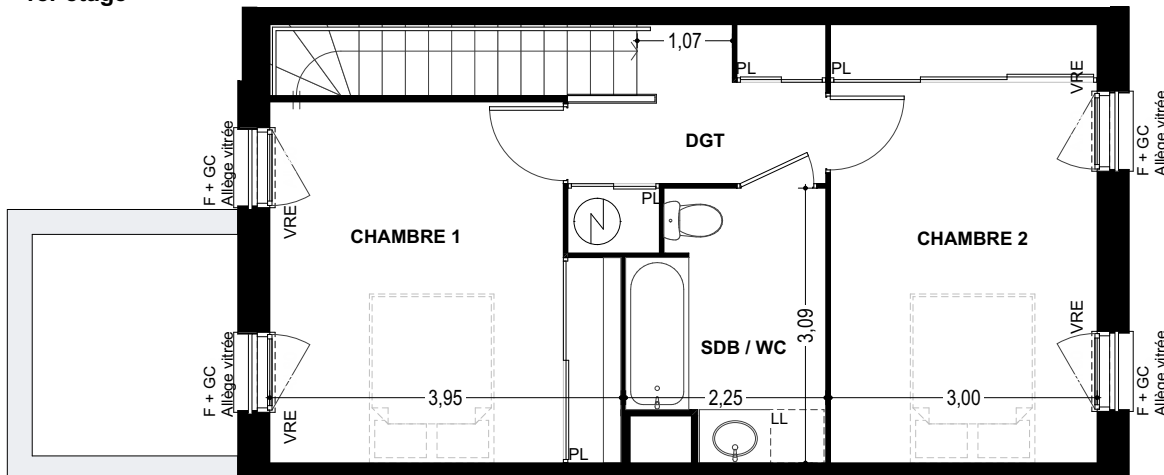
1er étage
