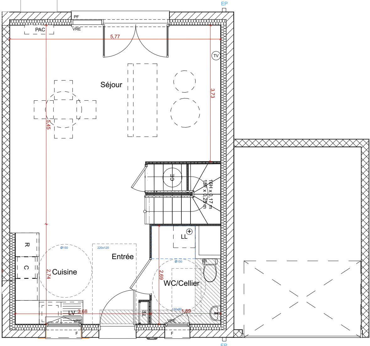
PLAN RdC
