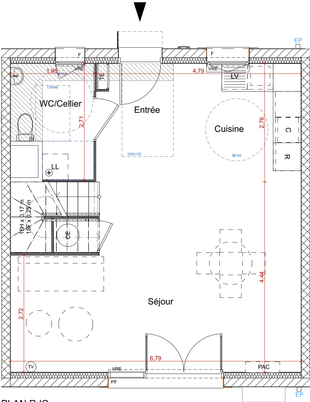
PLAN RdC
