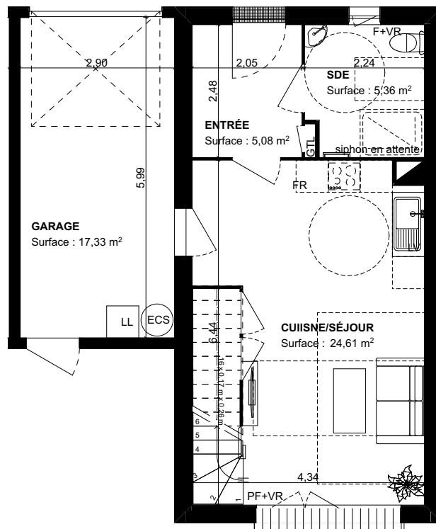
PLAN REZ DE CHAUSSEE
